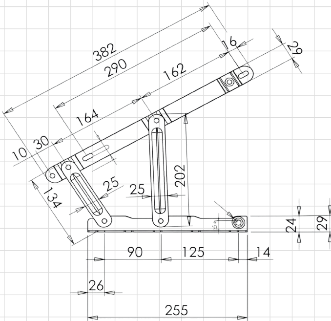
TST 4016 KÜÇÜK MEKANİZMA
